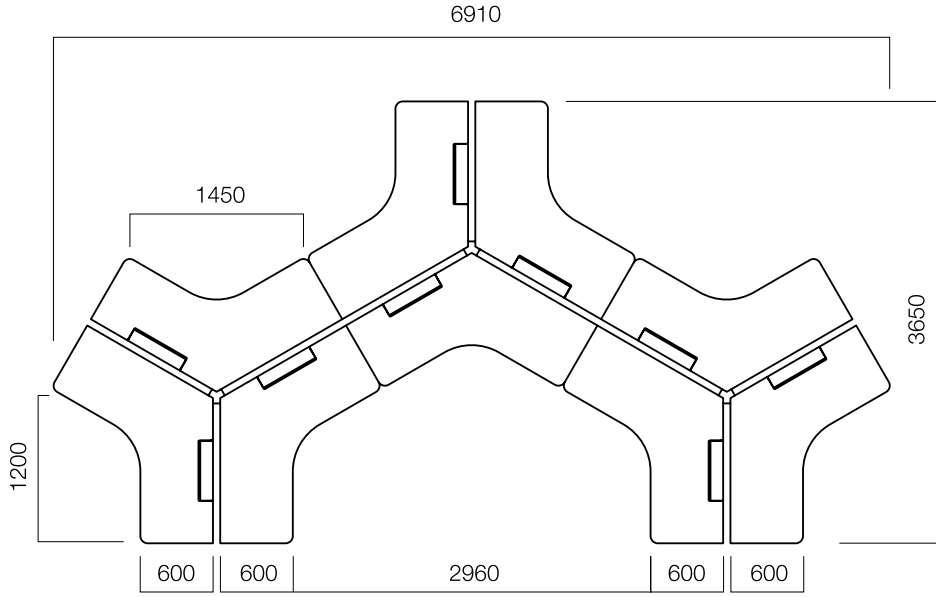
120° 9'lu Masa
