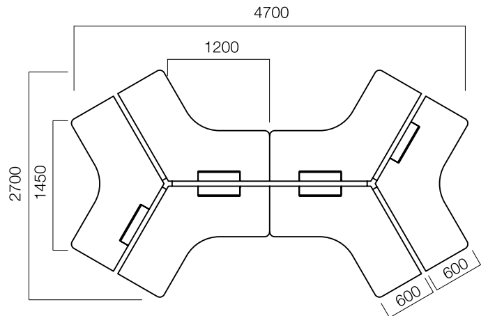
120° 6'lı Masa
