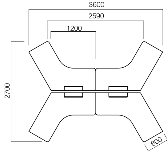
120° 4'lü Masa
