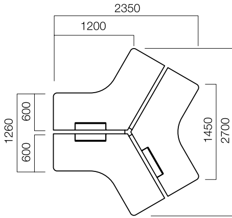
120° 3'lü Masa
