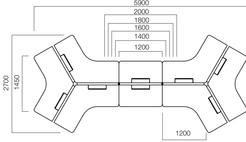
120° 8'li Masa
