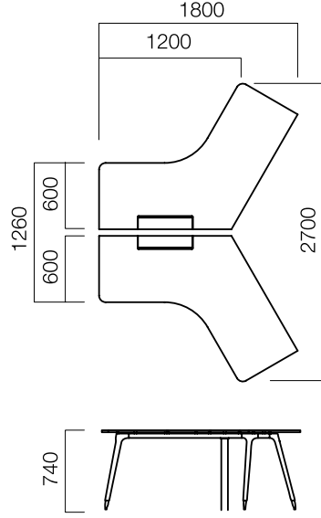
120° 2'li Masa
